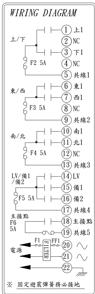
α 608A 接點圖 中文
