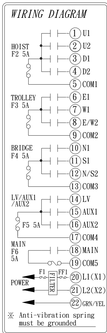
α 608B 接點圖 英文
