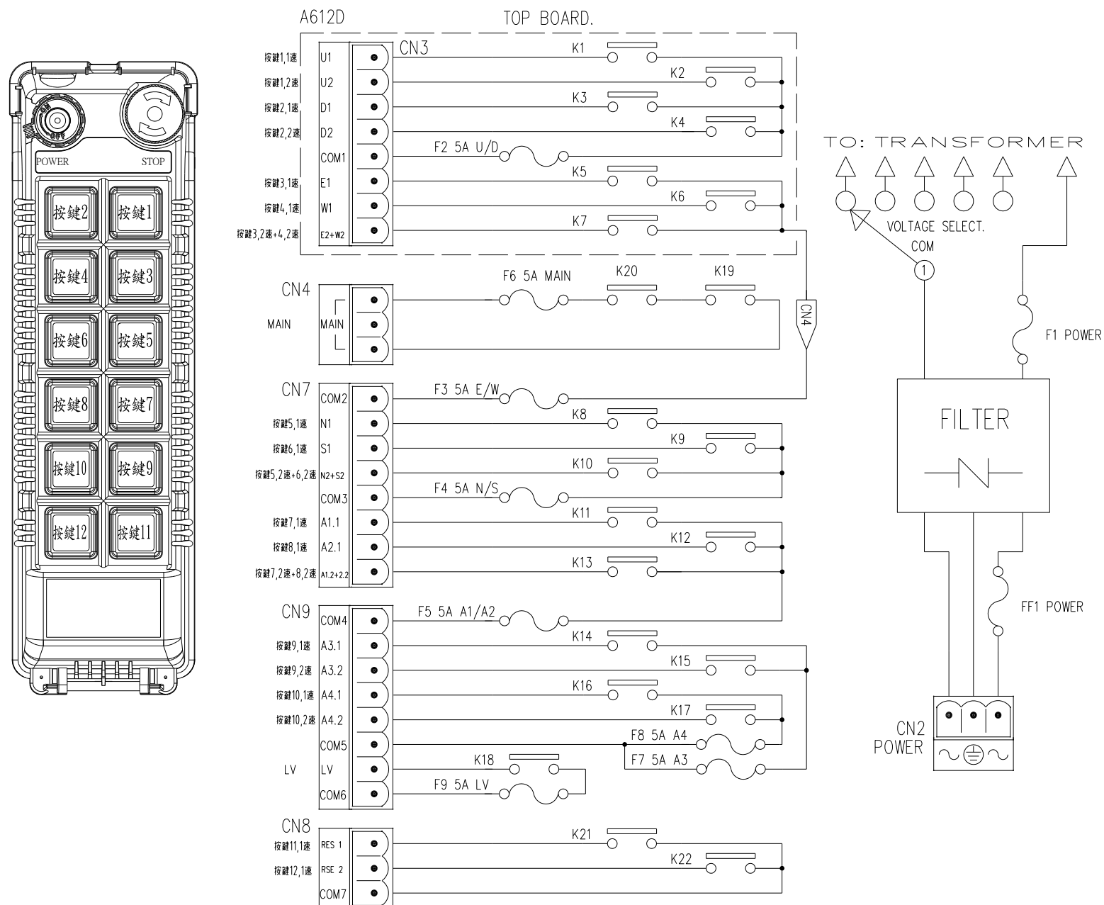
\alpha 612D 接收機接線圖
