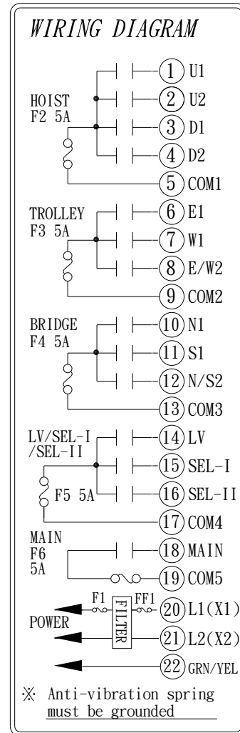
α 607BT 接點圖 英文
