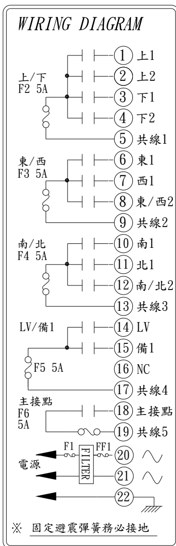
α 607B 接點圖 中文
