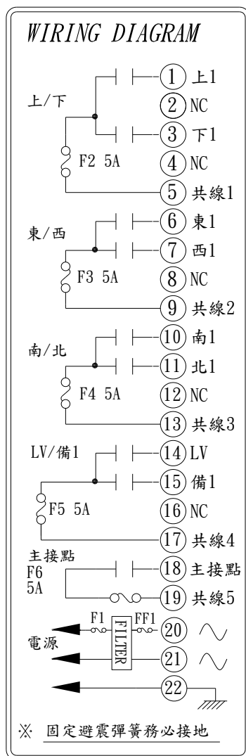
α 607A 接點圖 中文
