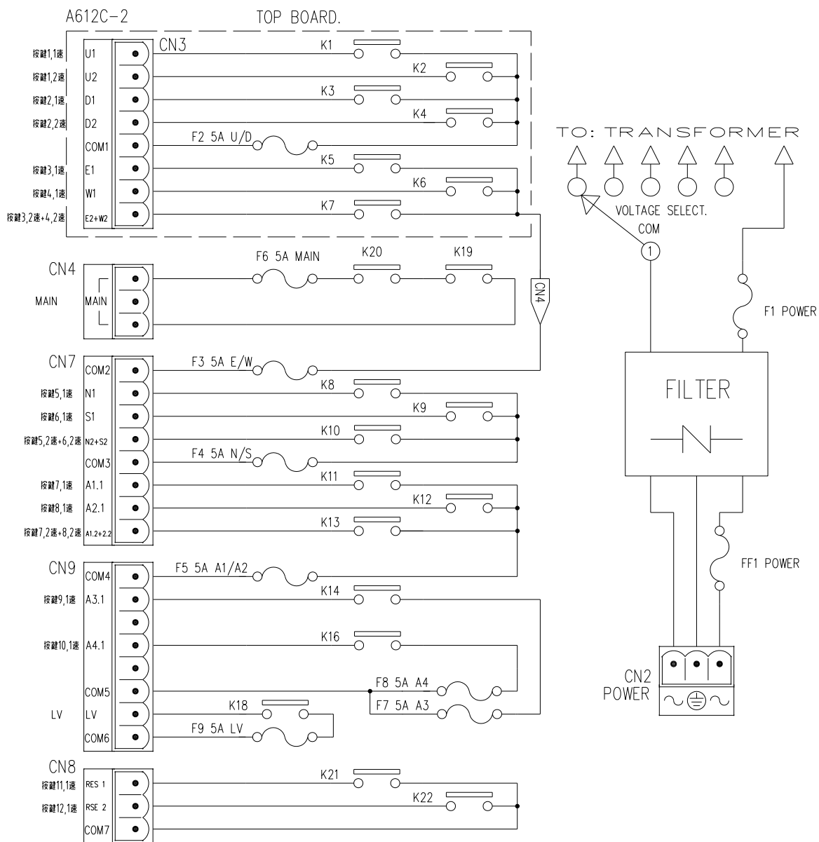
\alpha 612C-2 接收機接線圖
