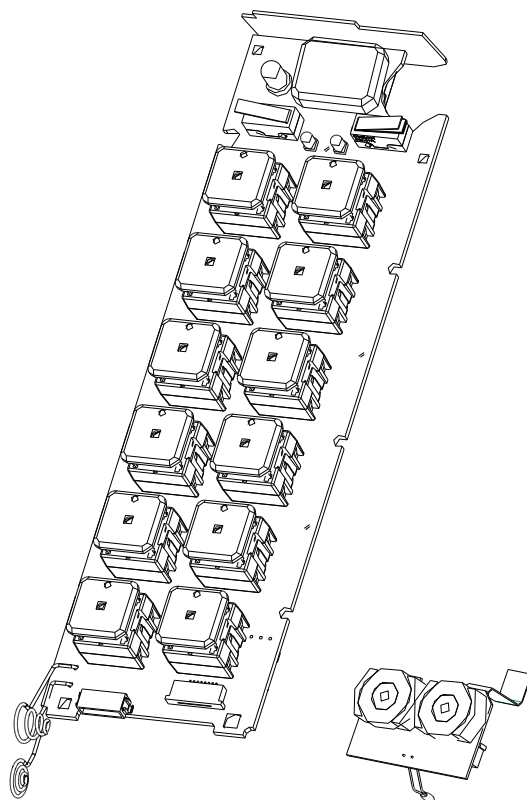
(1) 編碼發射板
