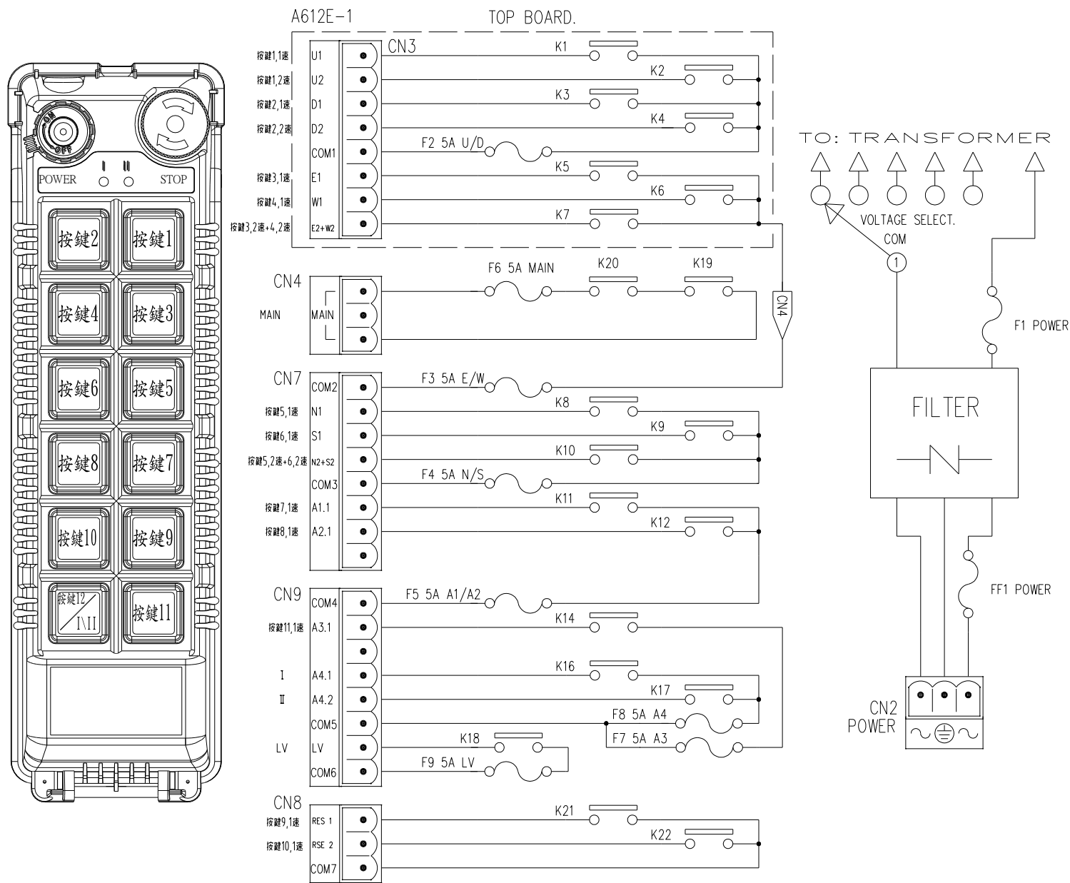
\alpha 612E-1 接收機接線圖
