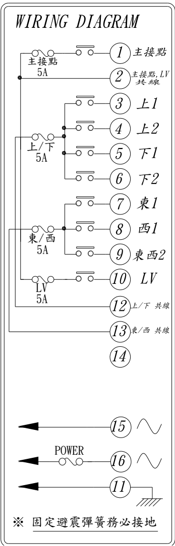
α 604B 接點圖 中文
