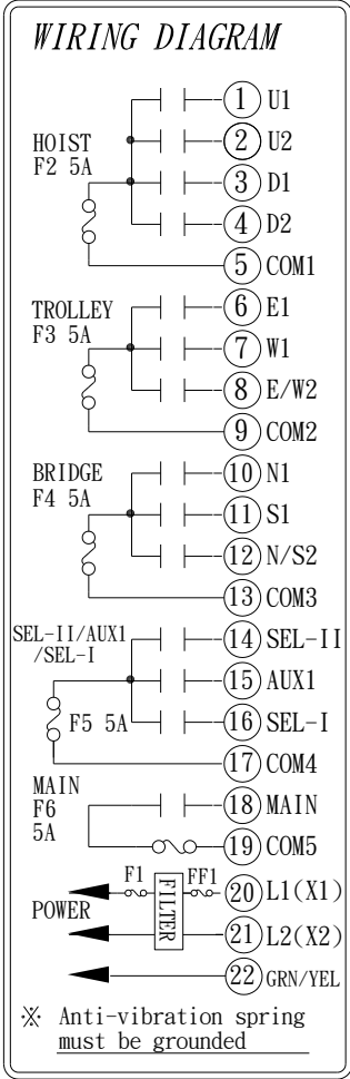
α 608BT 接點圖 英文
