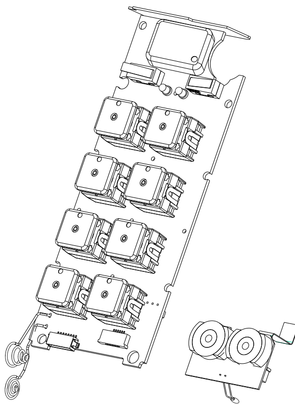
(1) 編碼發射板
