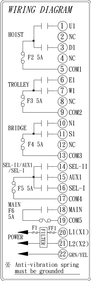
α 608AT 接點圖 英文
