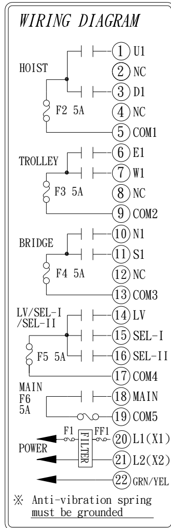
α 607AT 接點圖 英文
