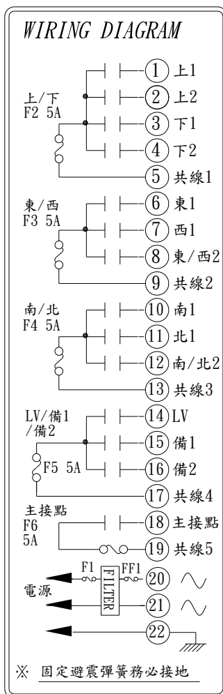
α 608B 接點圖 中文
