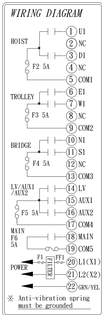
α 608A 接點圖 英文
