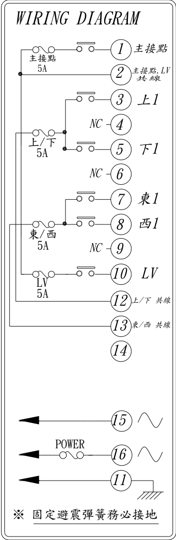
α 604A 接點圖 中文
